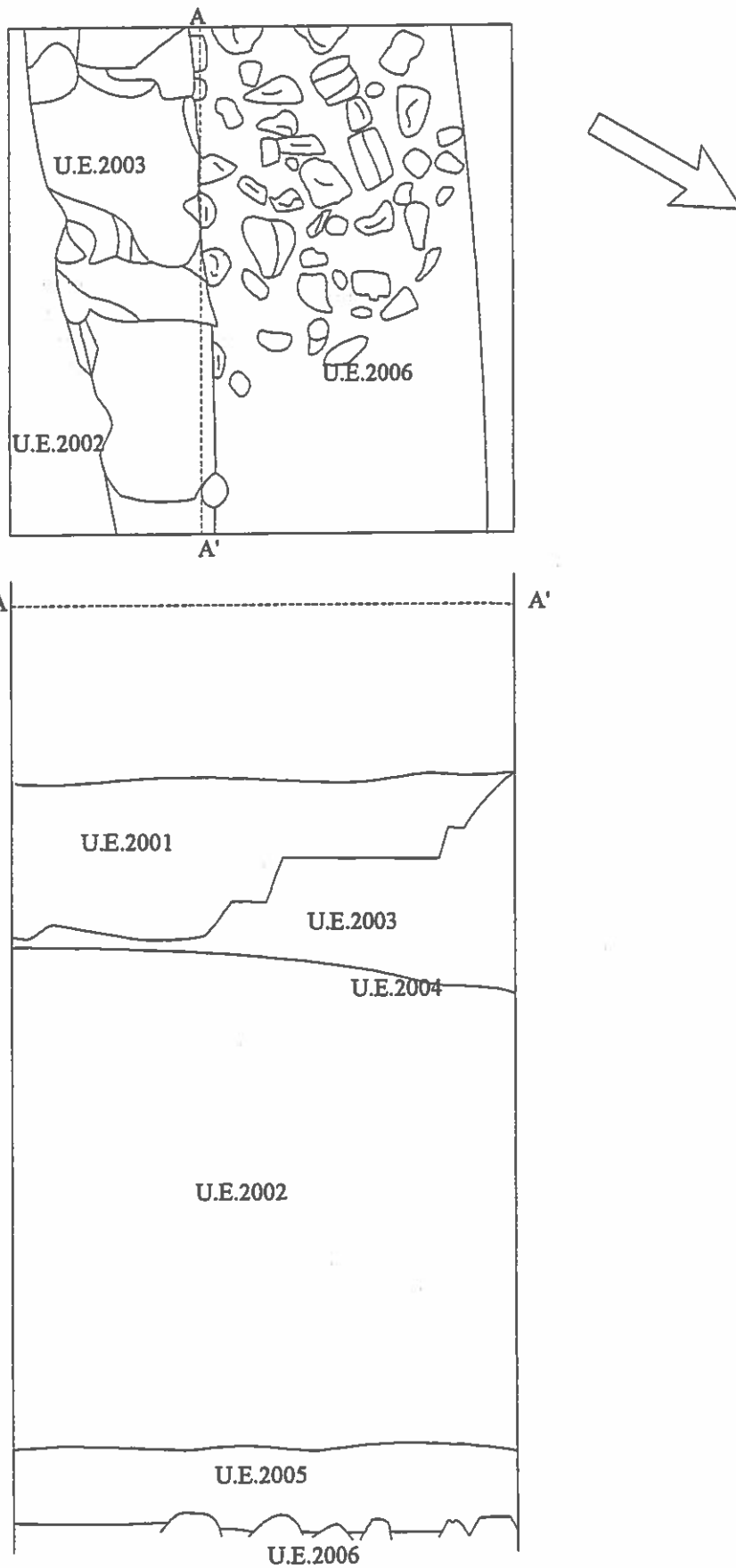
Fig.3: Planta i secció del sondeig Q.2 (E.1:20)
